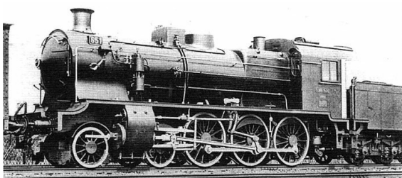
3 5 gekuppelte 2 Cylinder Heissdampf Personenzug-Locomotive der Sächsischen Staatsbahn. Ausgestellt zur Brüssler Weltausstellung 1910. Erbaut von der Sächsischen Maschinenfabrik vormals Rich. Hartmann, Chemnitz 1910.
